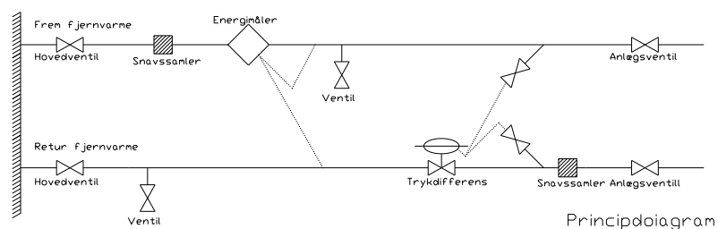
Principdiagram
